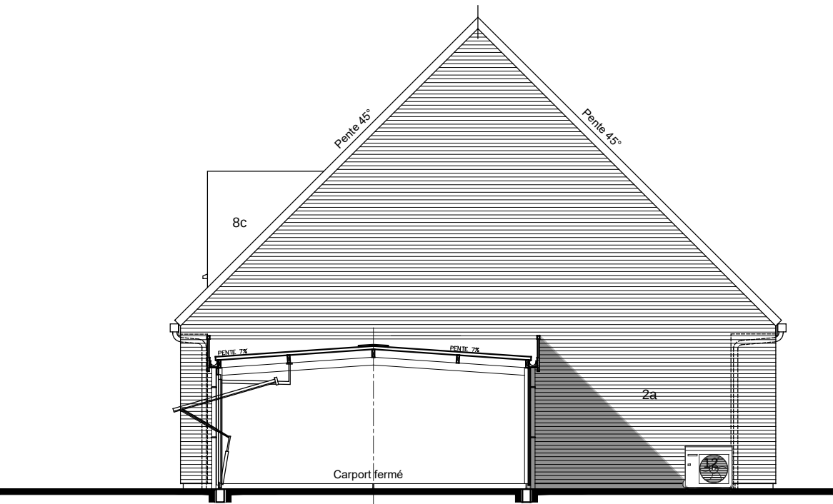
PIGNON DROIT
