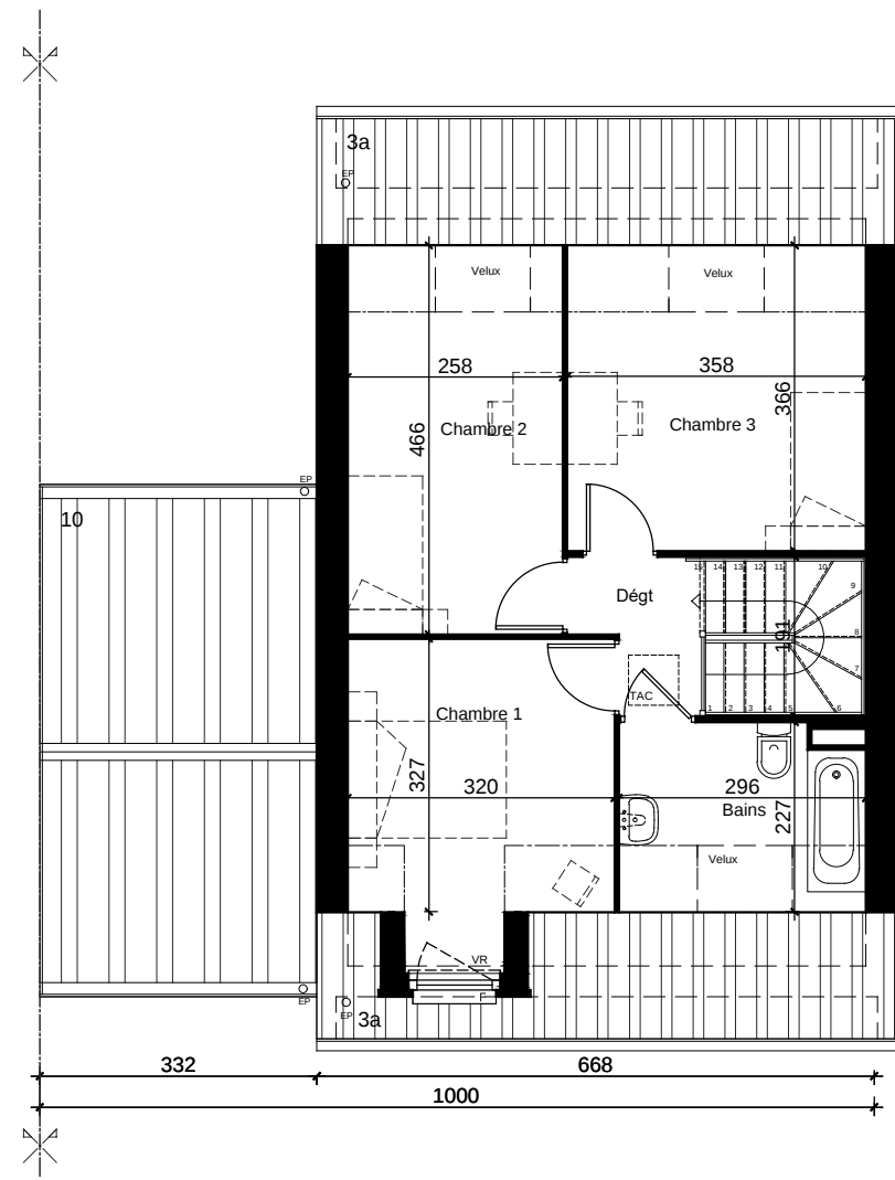
PLAN DU 1er ETAGE
