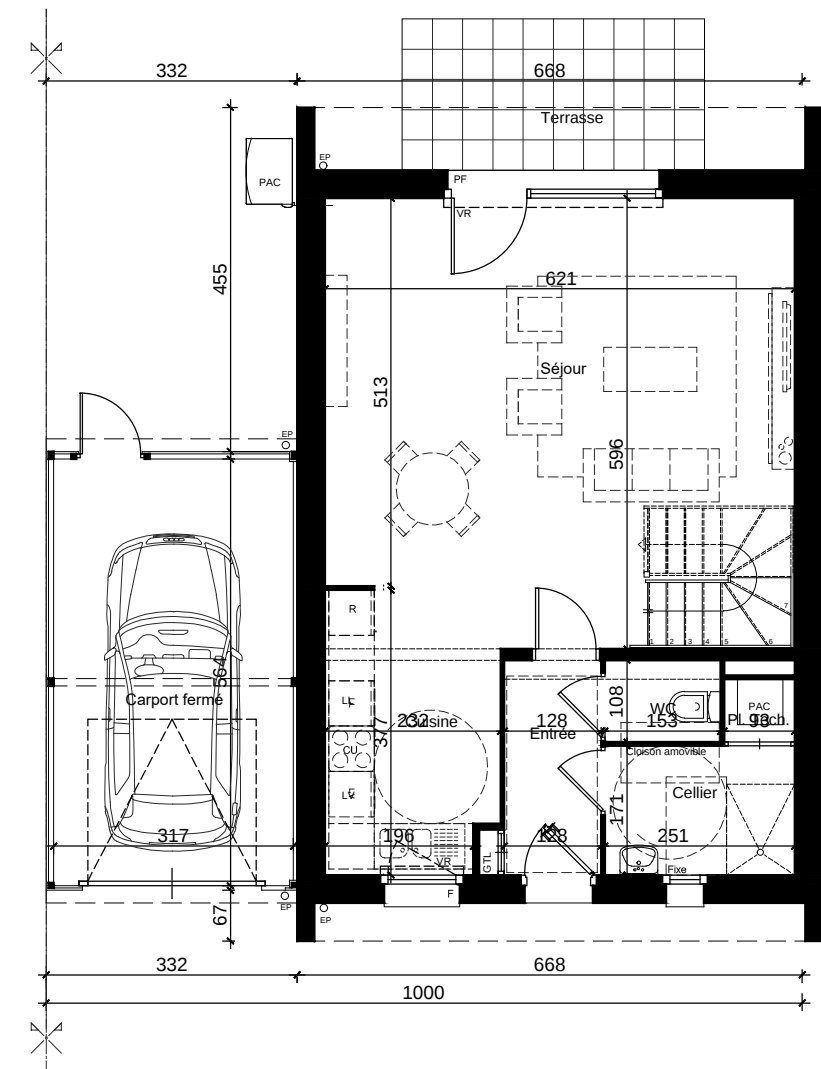
PLAN DE REZ DE CHAUSSEE
