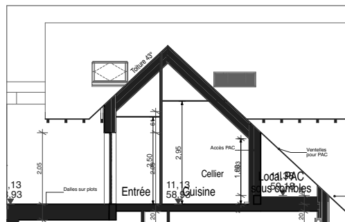
Coupe AA
