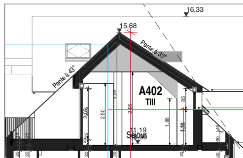
Coupe BB
