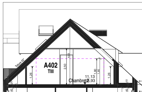
Coupe CC
