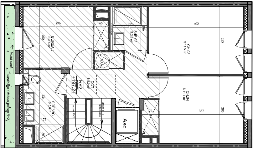
Plan de niveau R+2
