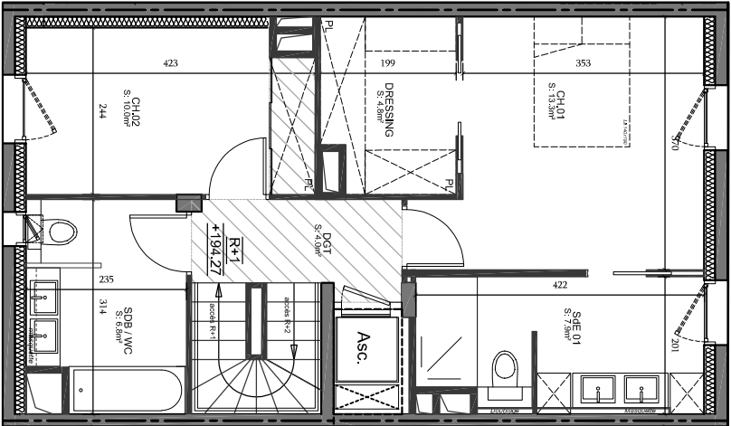
Plan de niveau R+1
