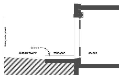
Coupe AA
